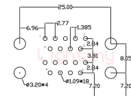
PCB布局 (PCB Layout)
