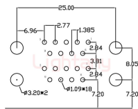
PCB布局 (PCB Layout)
