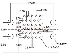
PCB布局 (PCB Layout)
