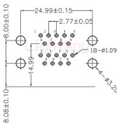
PCB布局 (PCB Layout)
